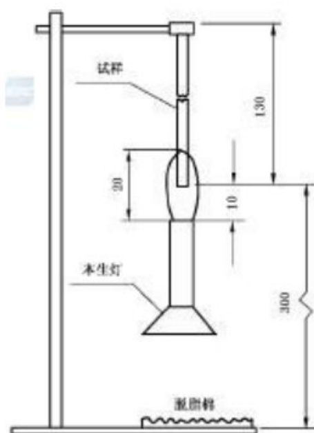
图 2 试验装置示意图
