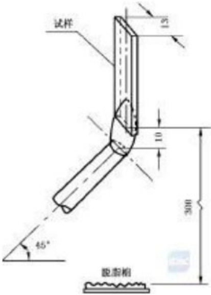
图 3 本生灯倾斜示意
